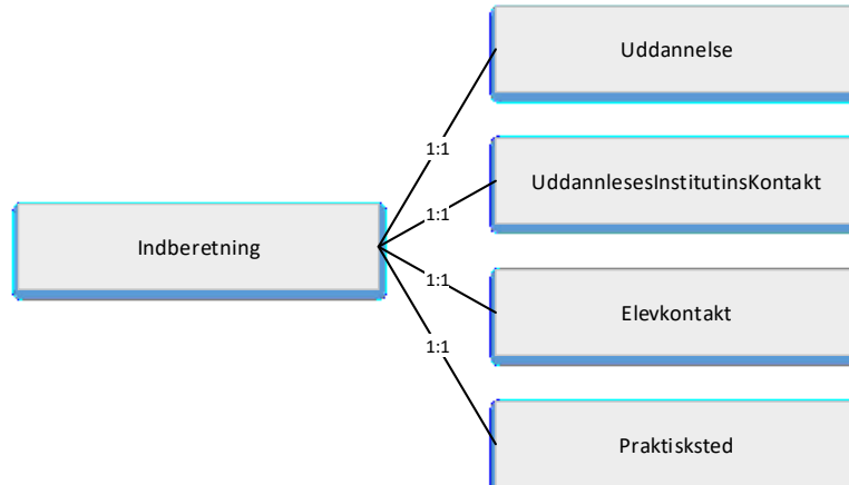
Figur 1: XML-struktur for IndberetUngdomsUddannelse.
