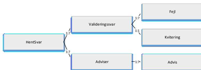
Figur 3: XML-struktur for afhentning af valideringssvar og adviseringer.
